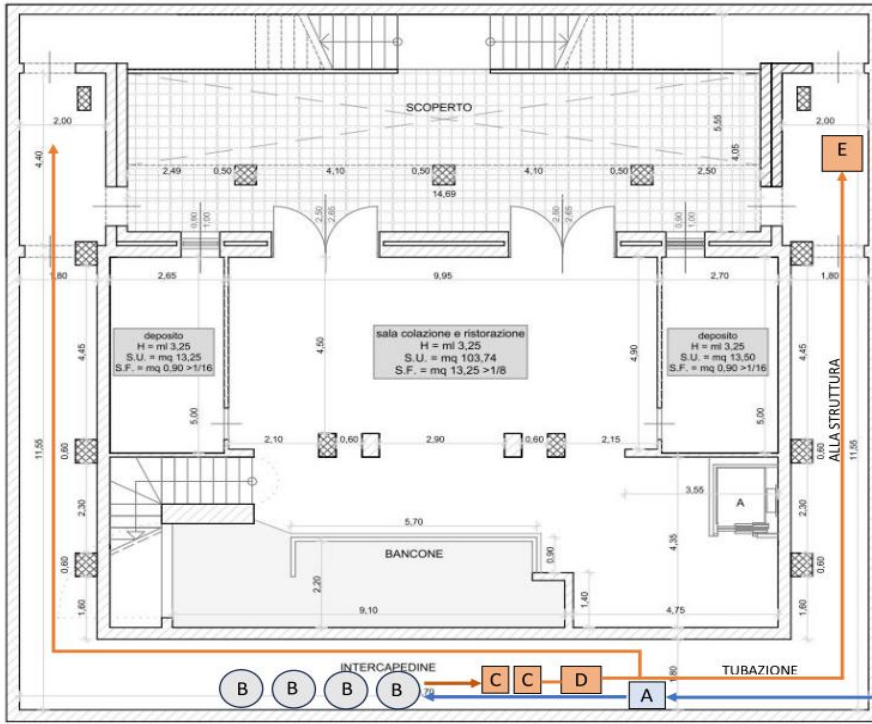
PIANTA PIANO INTERRATO - 1:100
