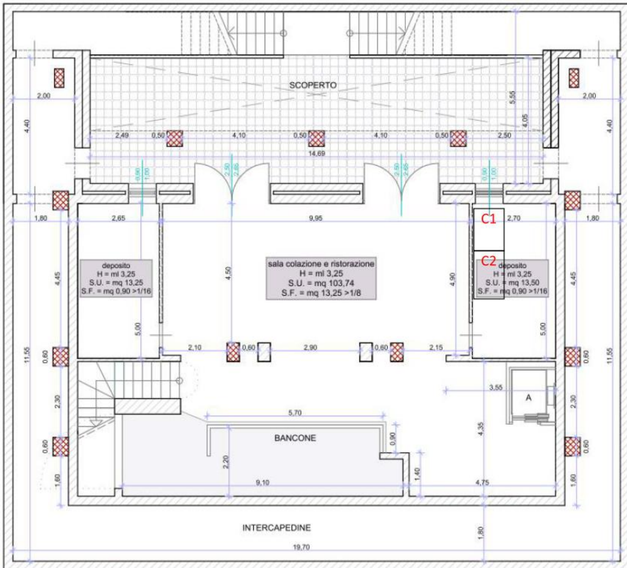
PIANTA PIANO INTERRATO - 1:100
