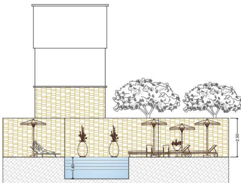
SEZIONE B-B IN VARIANTE
