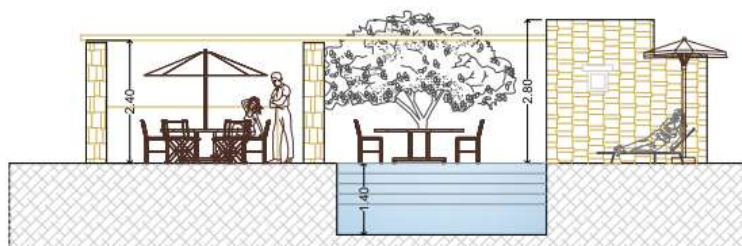
SEZIONE C-C IN VARIANTE
