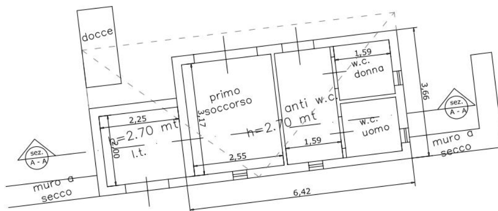
PIANTA SERVIZI PISCINA SC. 1:100
