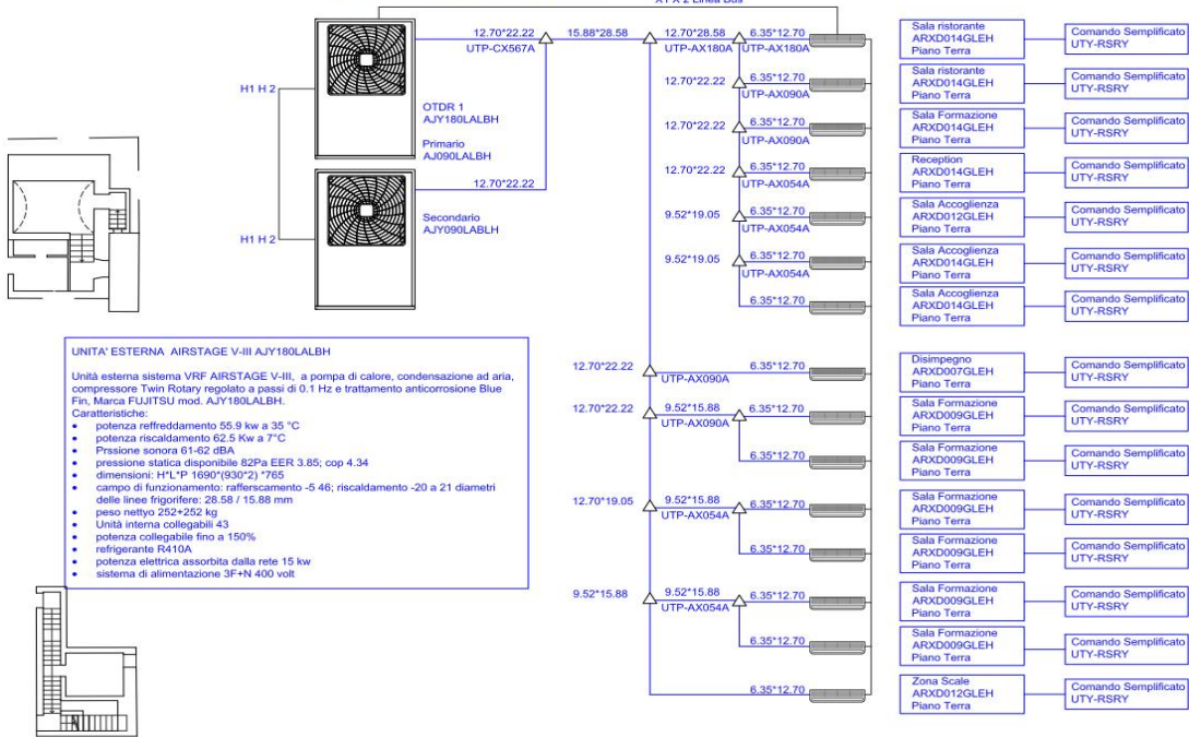
DIAGRAMMA TUBAZIONI OTDR 1 PIANO TERRA CONNESSIONE LOOP MACCHINE INTERNE/ESTERNE
