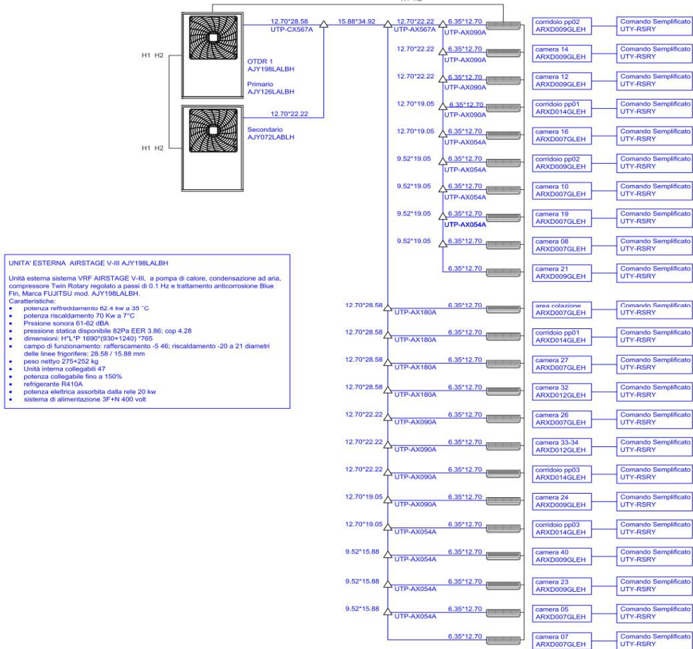
DIAGRAMMA TUBAZIONI OTDR 1 PIANO PRIMO CONNESSIONE LOOP MACCHINE INTERNE/ESTERNE
