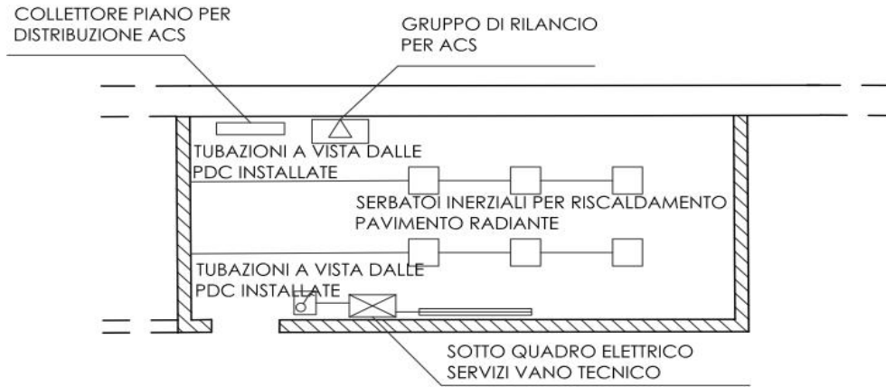
PIANTA VANO TECNICO
