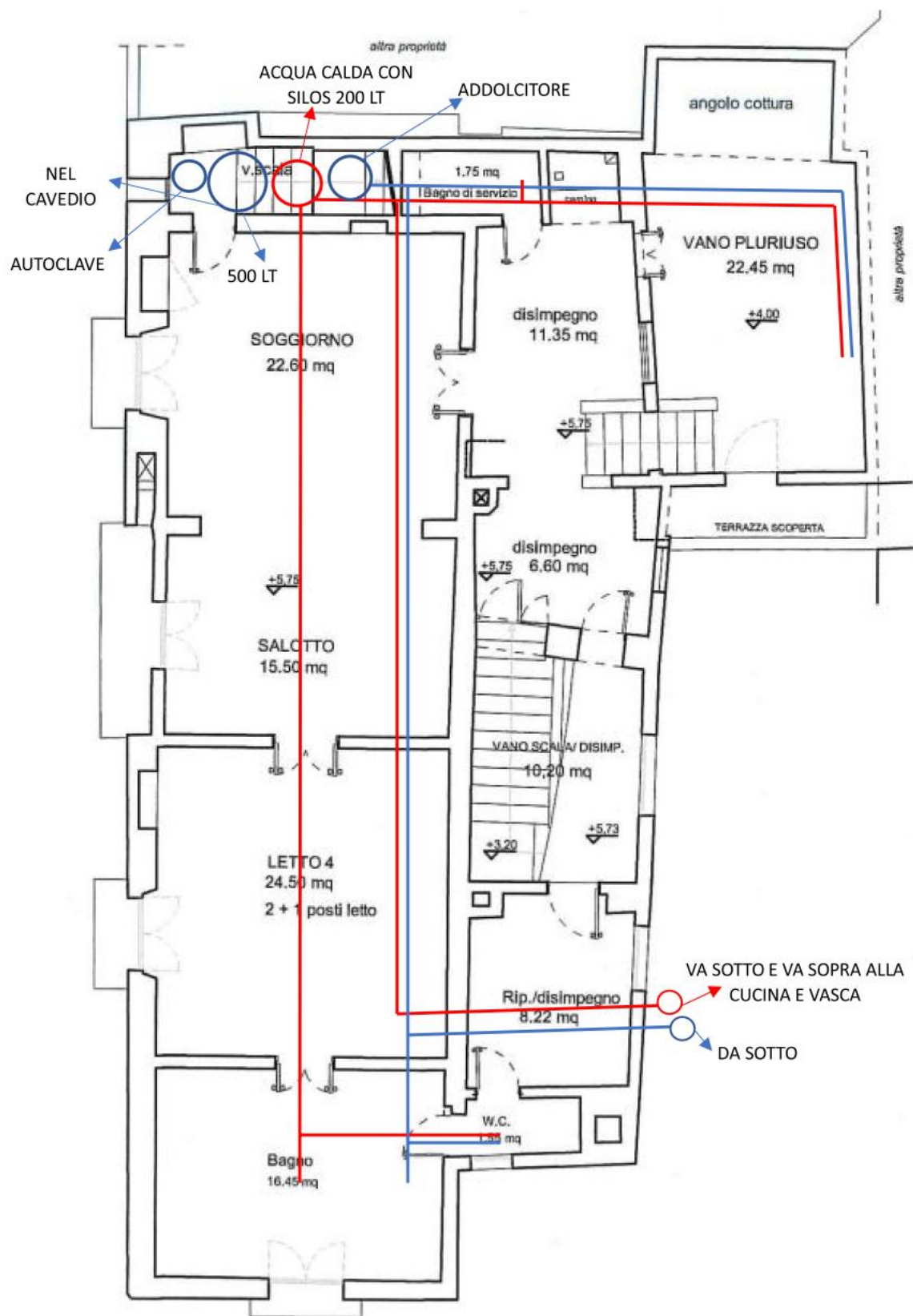
PIANO PRIMO - scala 1:100
