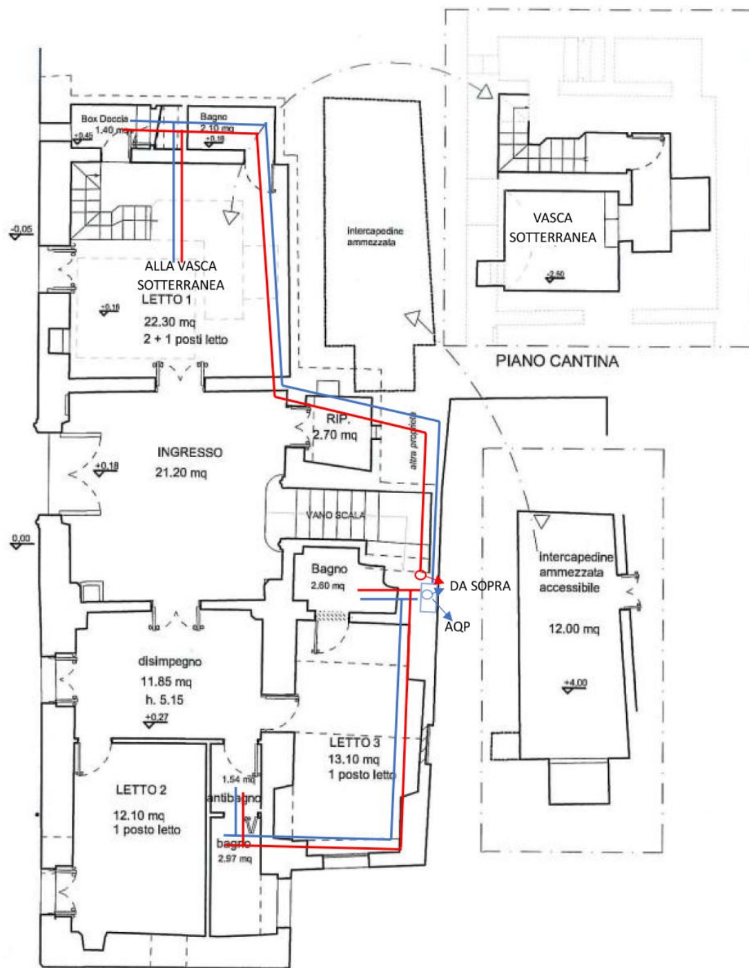
PIANO TERRA - scala 1:100
