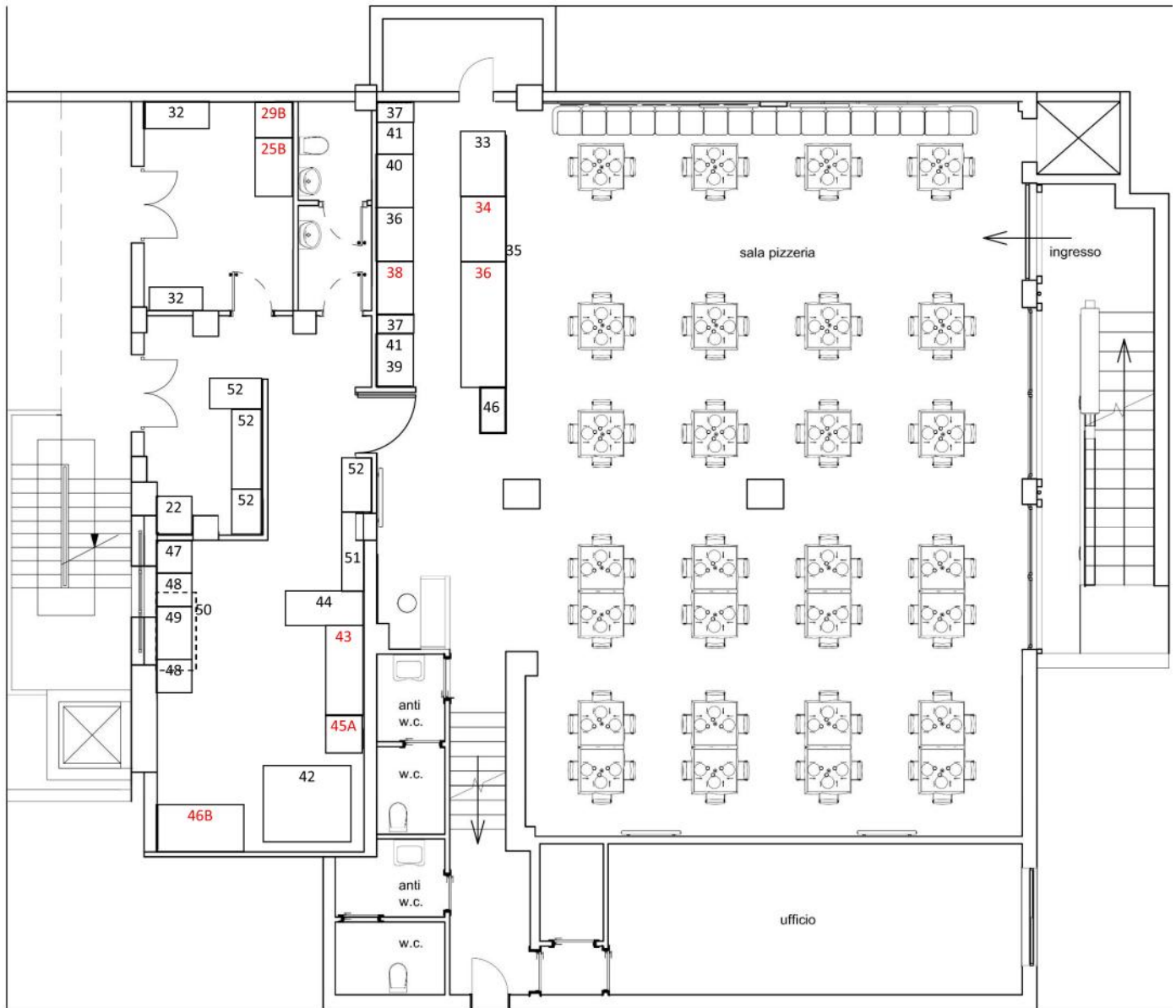
PLANIMETRIA GENERALE - PIANO SEMINTERRATO
